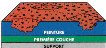
1- La peinture est soigneusement nettoyée pour enlever les salissures.
